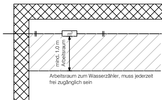
Grundriss
