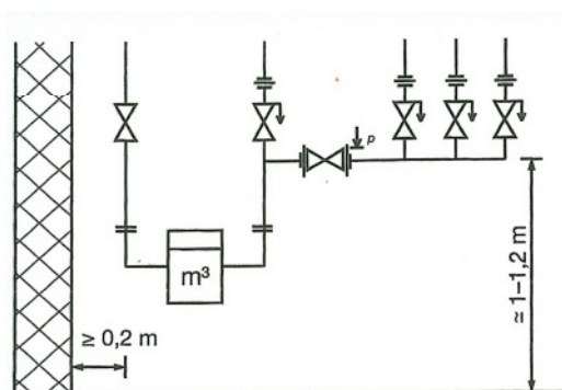
Ansicht
